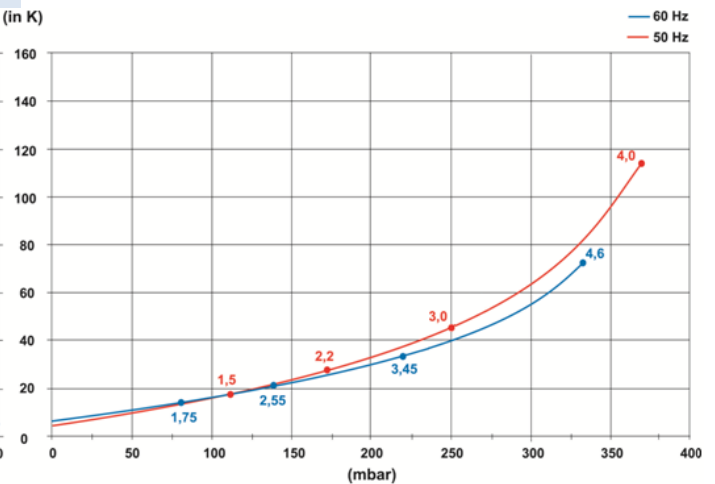
Förderlufterwärmung / Temperature rise on the exhaust air
