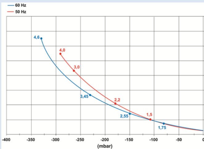
Förderlufterwärmung / Temperature rise on the exhaust air
